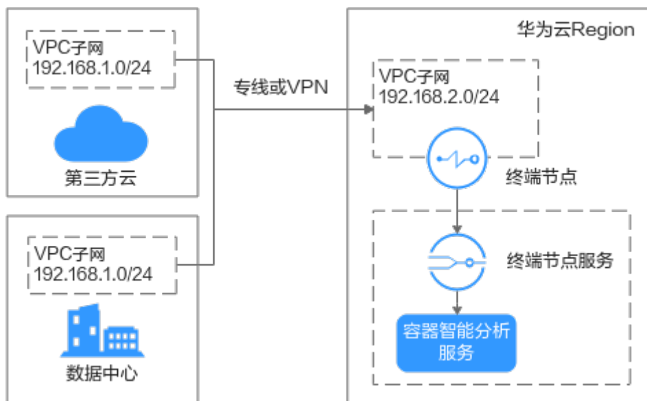
图 6-2 私网接入原理
