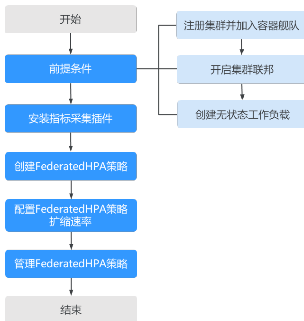
图 3-29 FederatedHPA 使用流程
