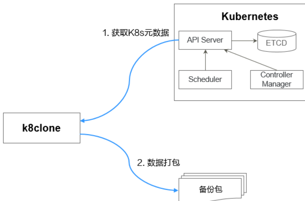
图 9-17 数据备份流程
