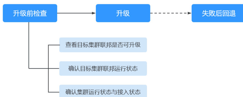
图 3-11 联邦升级流程
