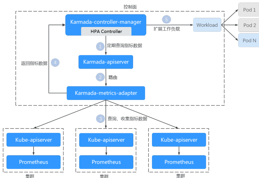
图 3-32 FederatedHPA 工作原理
