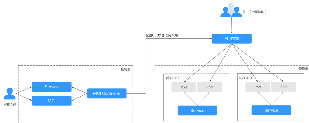
图 3-20 MCI Controller 工作原理
