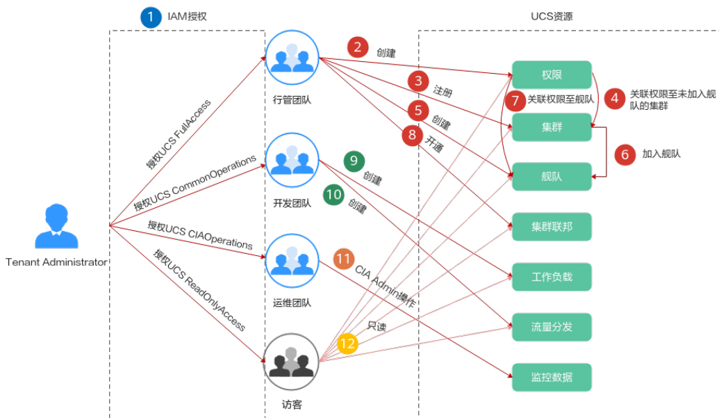
图 13-10 UCS 资源操作全景
