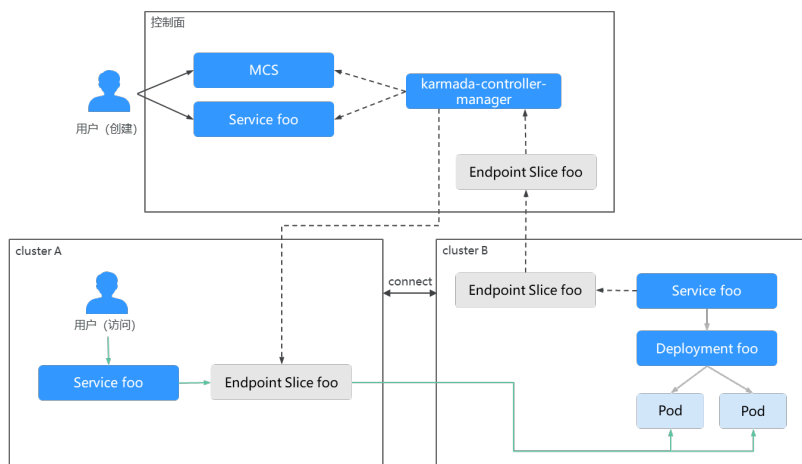
图 3-21 MCS 工作原理
