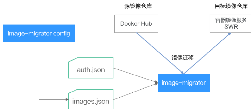
图 9-3 image-migrator 工作原理
