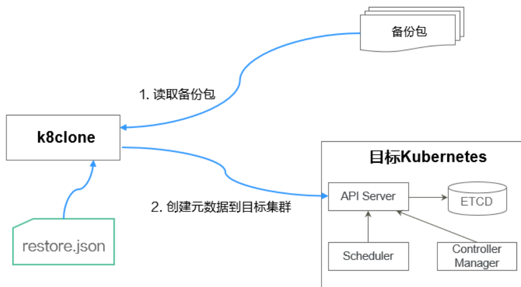
图 9-5 数据恢复流程
