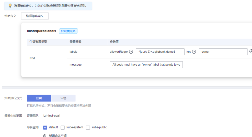
图 10-2 创建策略实例
