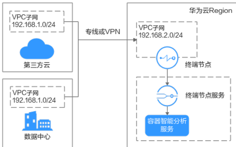
图 6-4 私网接入原理
