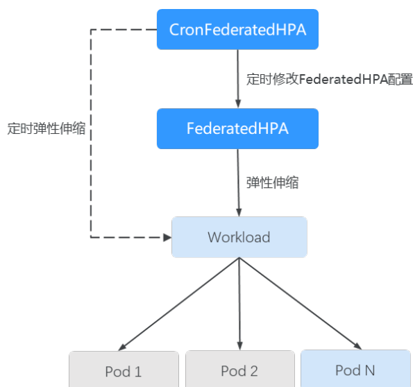
图 3-33 CronFederatedHPA 工作原理
