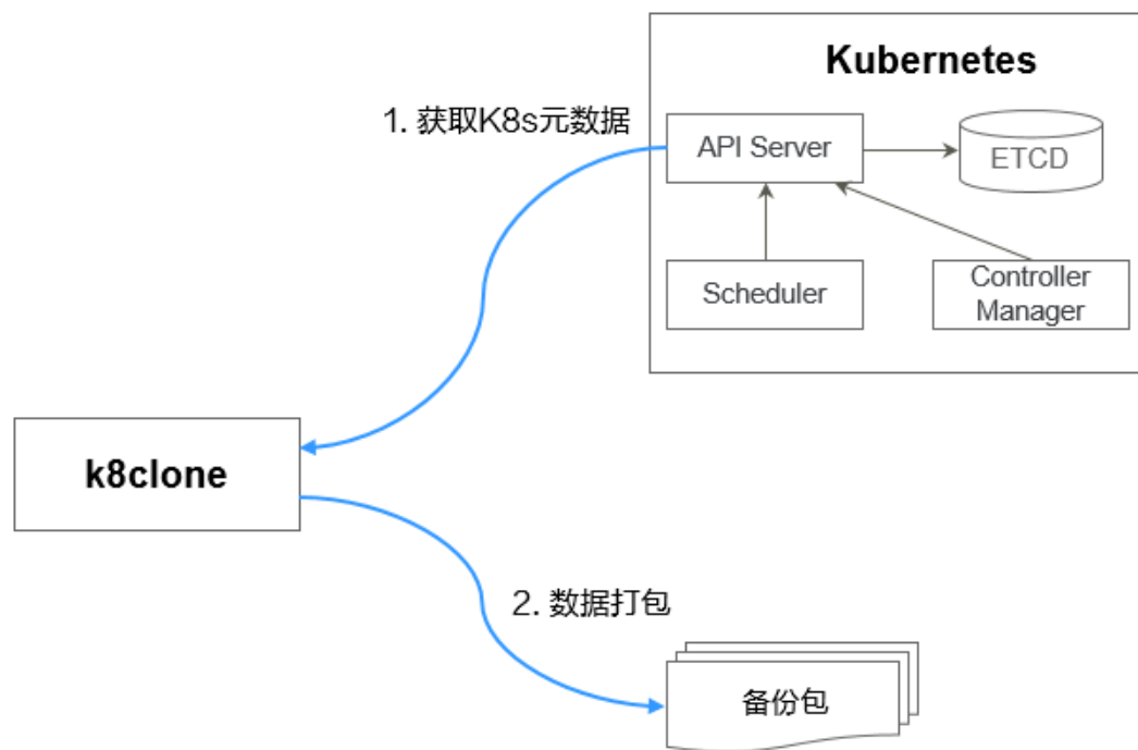
图 9-13 数据备份流程
