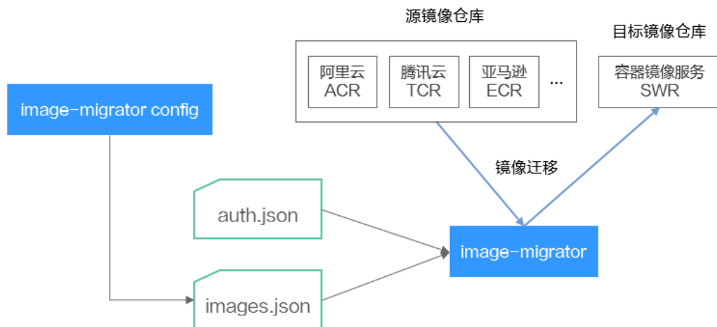
图 9-8 image-migrator 工作原理
