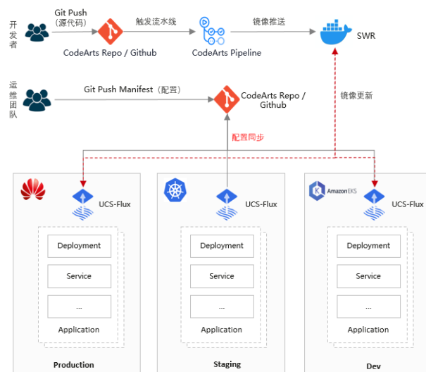
图 11-1 GitOps 实现方式
