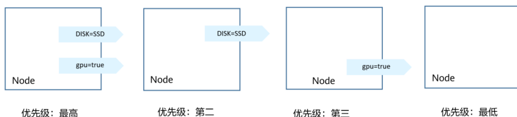
图 3-18 优先级排序顺序
