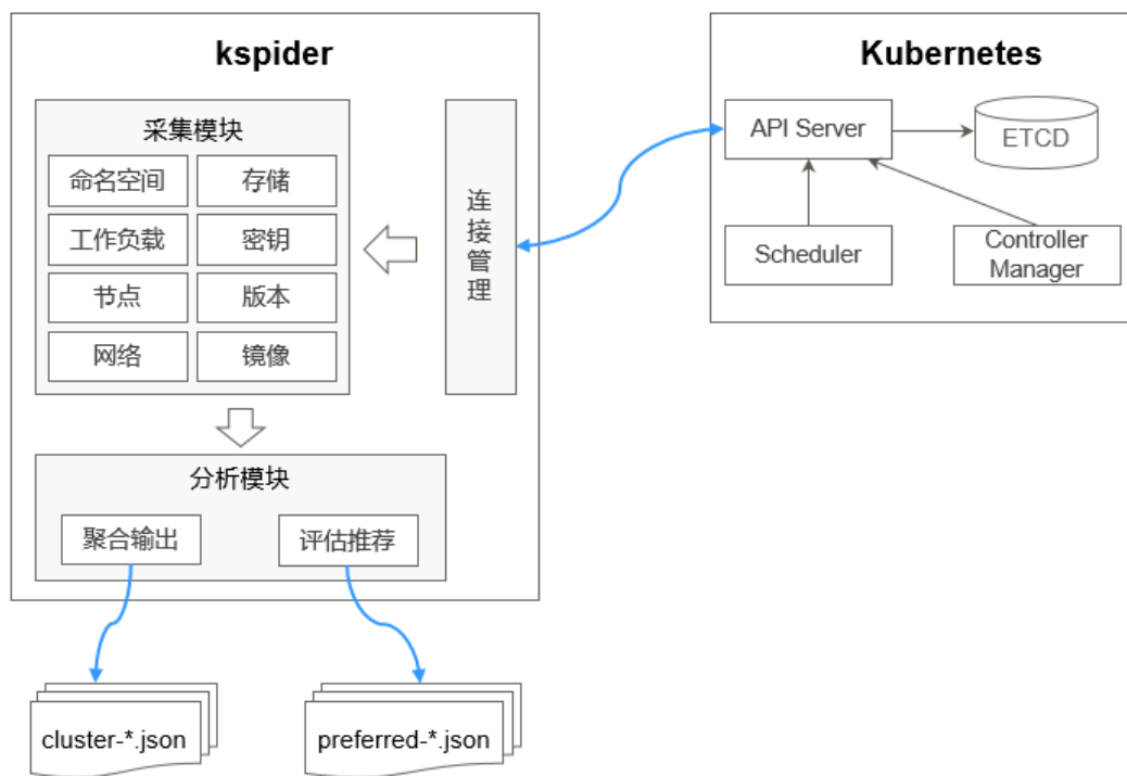
图 9-2 kspider 架构
