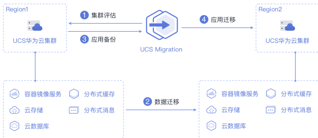
图 9-11 迁移流程
