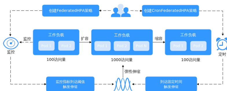
图 3-28 负载伸缩策略机制
