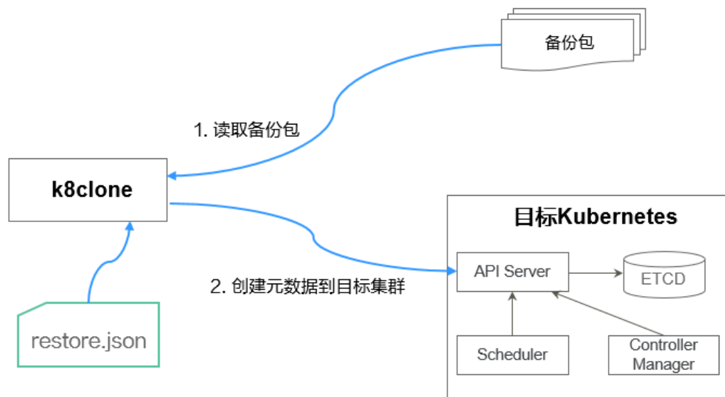
图 9-18 数据恢复流程
