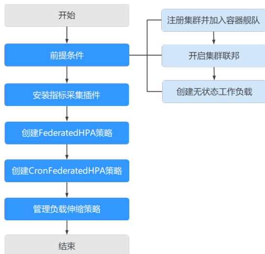
图 3-31 CronFederatedHPA 与 FederatedHPA 配合使用流程
