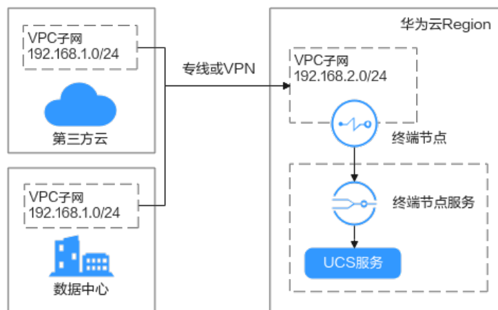
图 1-22 私网接入原理
