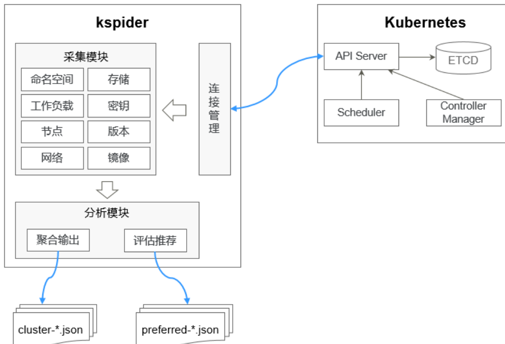
图 9-7 kspider 架构
