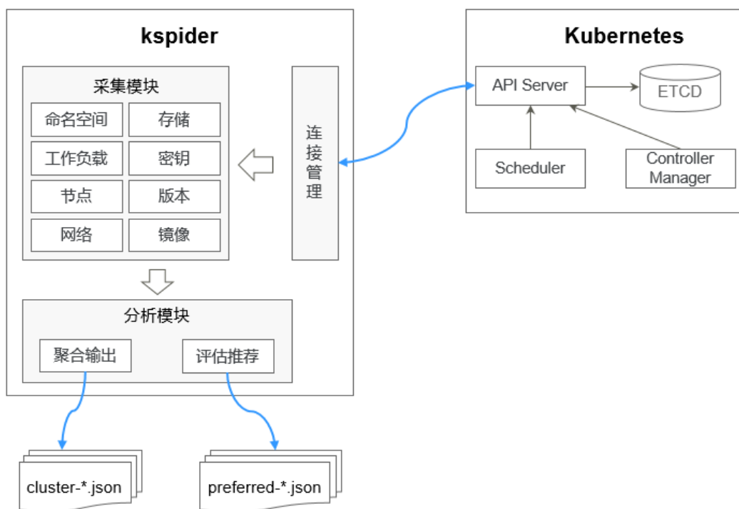
图 9-12 kspider 架构
